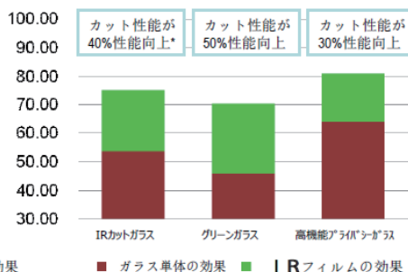
各ガラスにIRフィルムを貼った場合の IR Cut%
