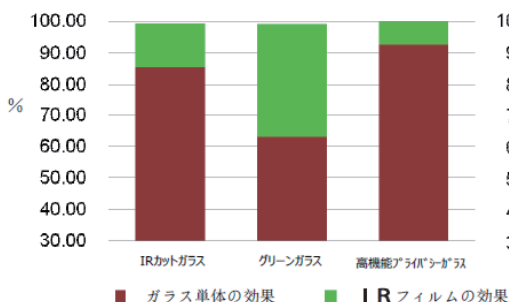
各ガラスにIRフィルムを貼った場合の UV Cut%
